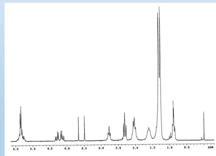
SPETTRO HNMR
