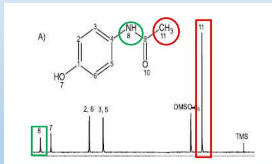
SPETTRO HNMR-PARACETAMOLO
